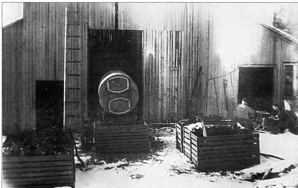
En retorter står på kylning innan den ska tömmas på kol.
